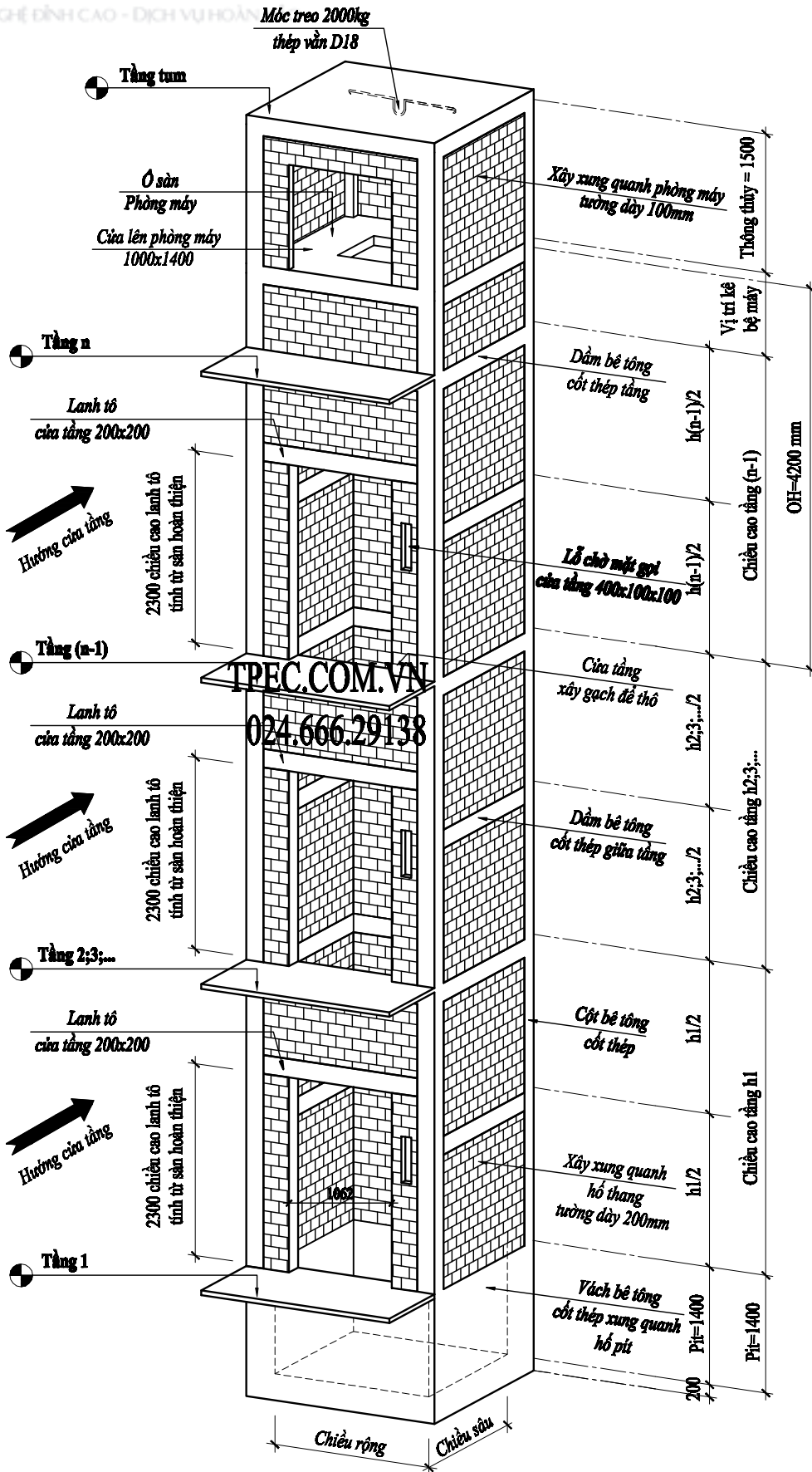
BẢN VẼ THANG MÁY - (CÓ PHÒNG MÁY)
