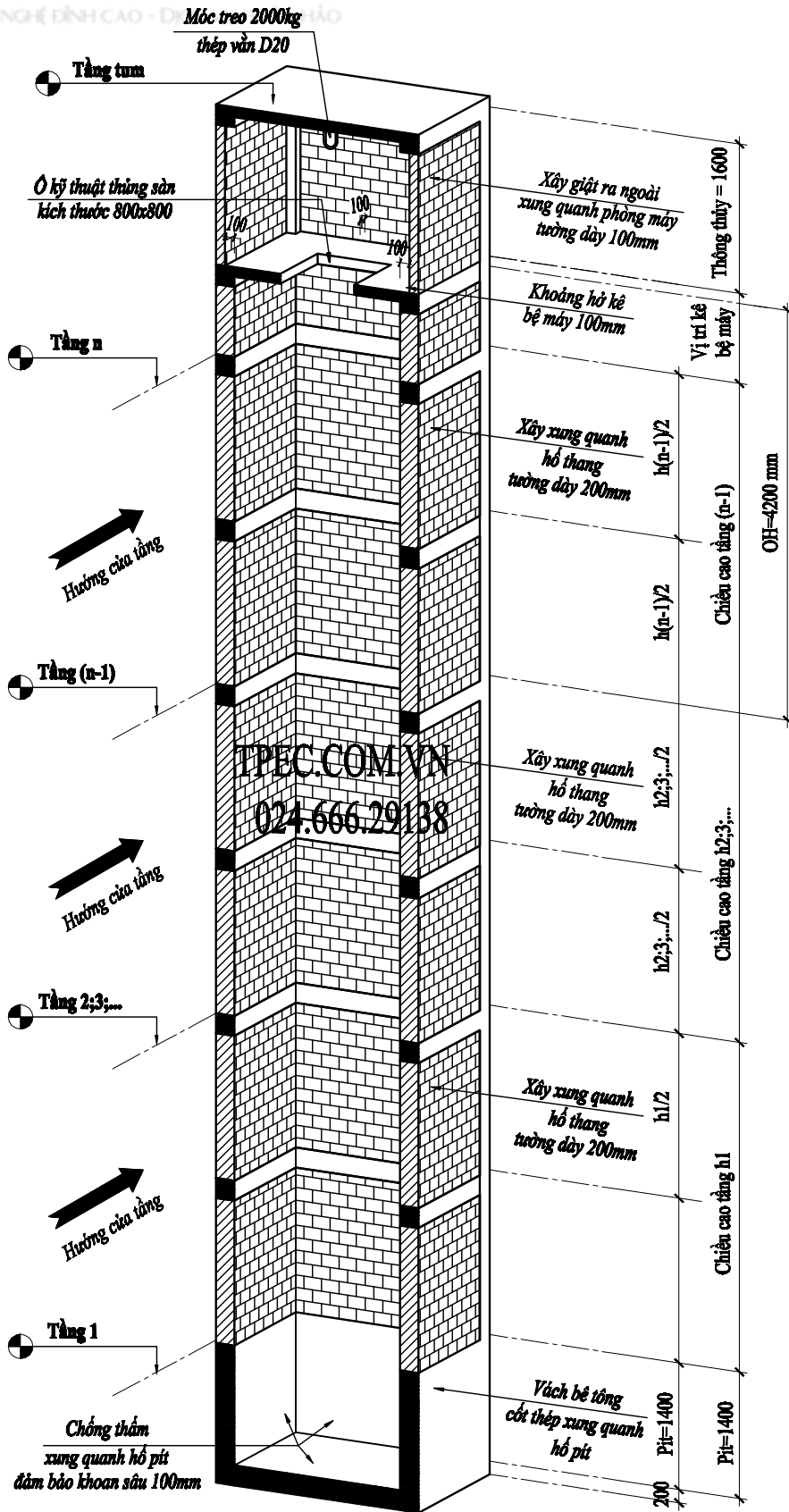
BẢN VẼ MẶT CẮT DỌC HỐ THANG MÁY - (CÓ PHÒNG MÁY)
