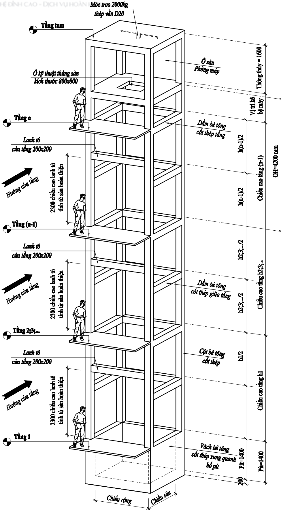
KHUNG KẾT CẤU HỒ THANG MÁY - (CÓ PHÒNG MÁY)
