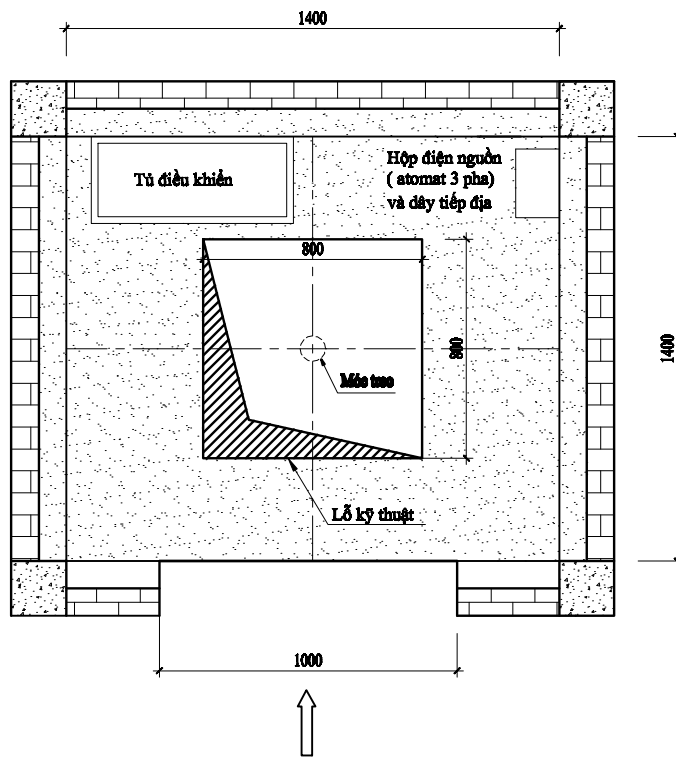
HƯỚNG CỬA PHÒNG MÁY RỘNG 1000; CAO >1500MM
