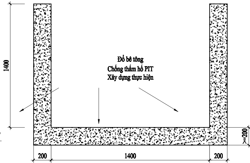
MẶT CẮT ĐỨNG HỒ PÍT HAI VÁCH HÔNG
