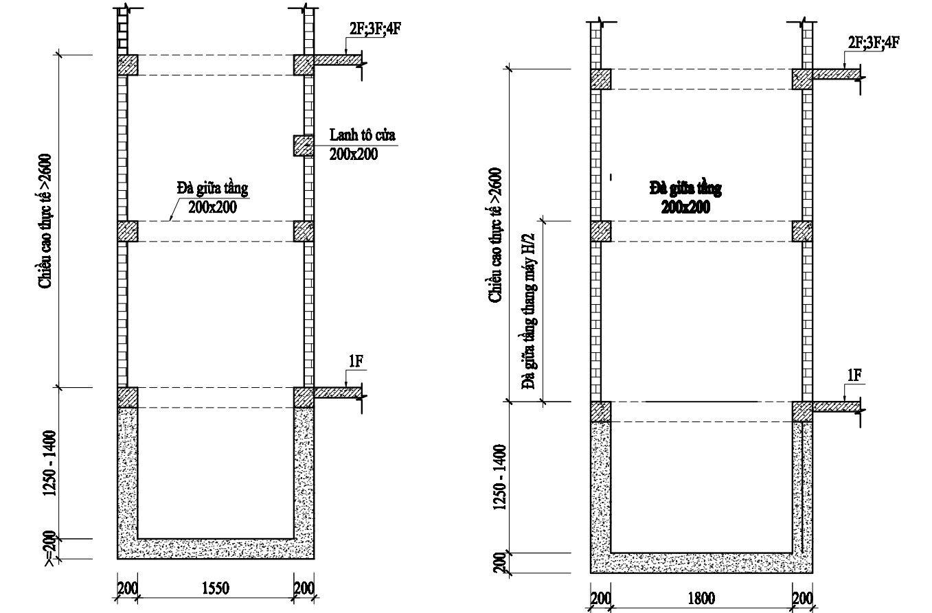
MẶT CẮT DỌC 2 BÊN HÔNG
