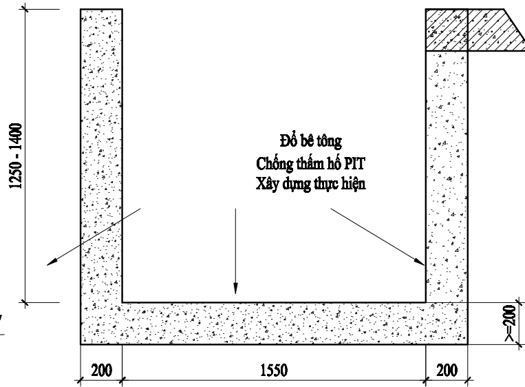
MẶT CẮT ĐỨNG HỒ PIT HAI VÁCH HÔNG
