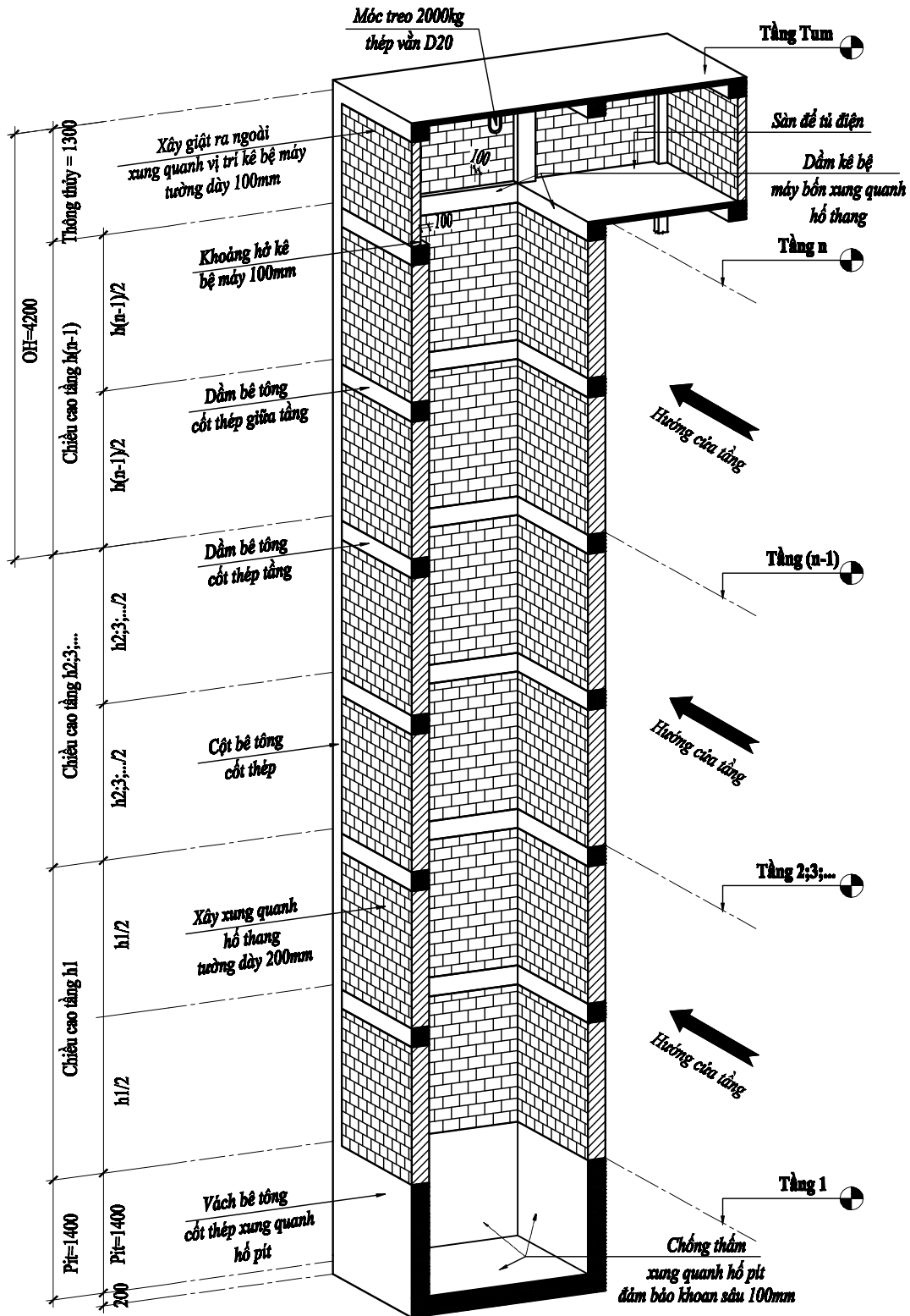
BẢN VẼ MẶT CẮT DỌC HỐ THANG MÁY - ( KHÔNG PHÒNG MÁY )
