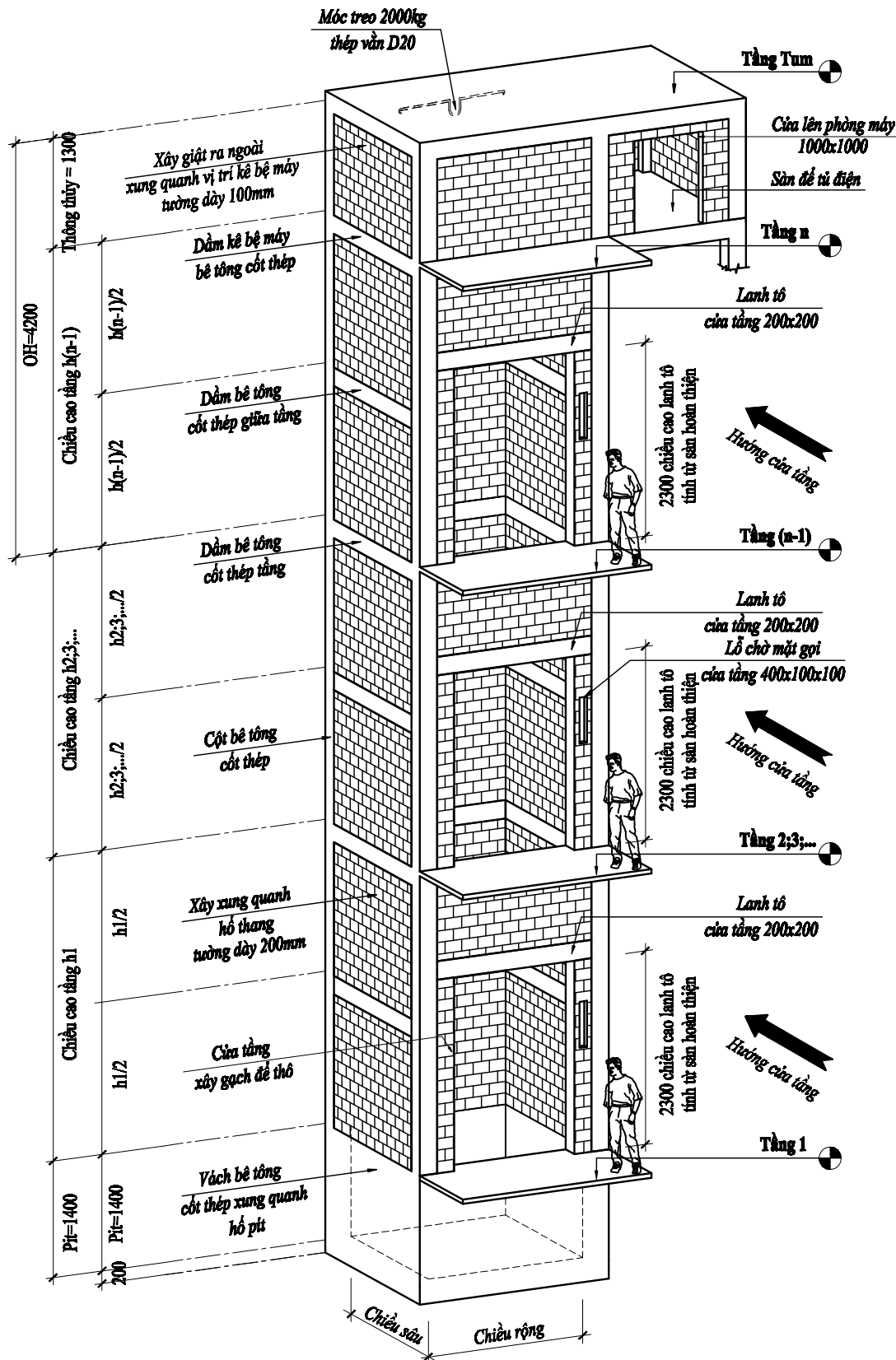
BẢN VẼ THANG MÁY - (KHÔNG PHÒNG MÁY)
